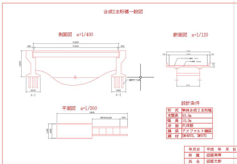
図2 AutoCAD で作成した図面
