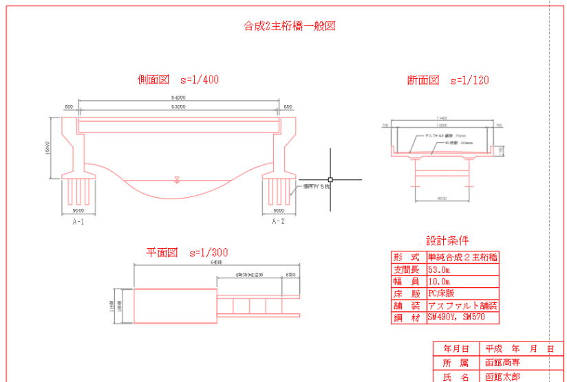
図2 AutoCAD で作成した図面
