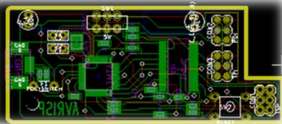
図 1 CAD 画面
